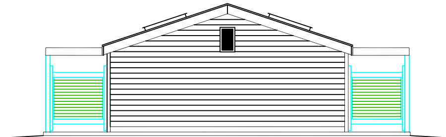
END ELEVATION
