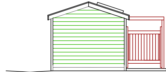
LEFT ELEV.
